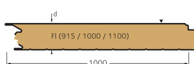
Stěnový panel – skrytý spoj PFLAUM FI
